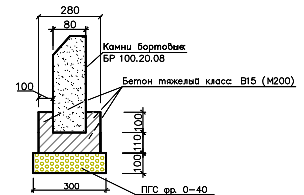
Узел бортового камня БР 100.20.8
